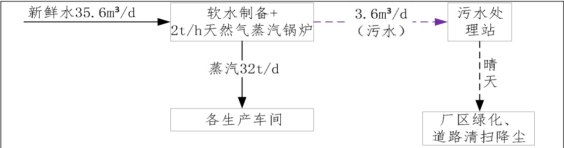
图 2.2.2-1 本项目建成后锅炉房水量平衡图
