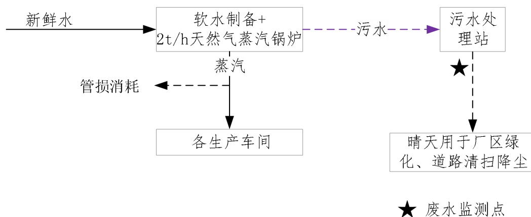
图 3.2-1 项目废水流向图
