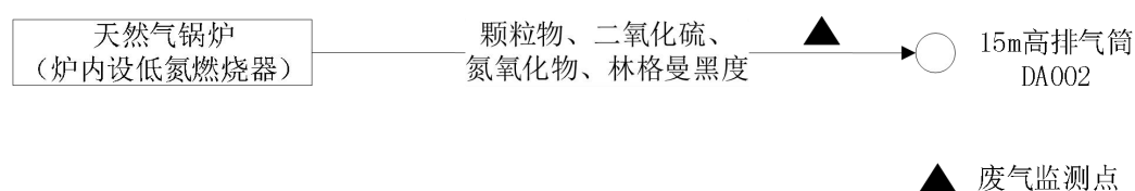
图 3.3-1 项目锅炉废气流向图
