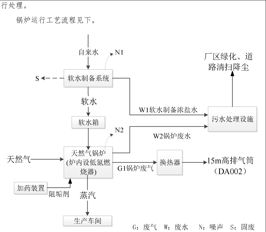
图 2.3-1 生产工艺流程及产污环节图
