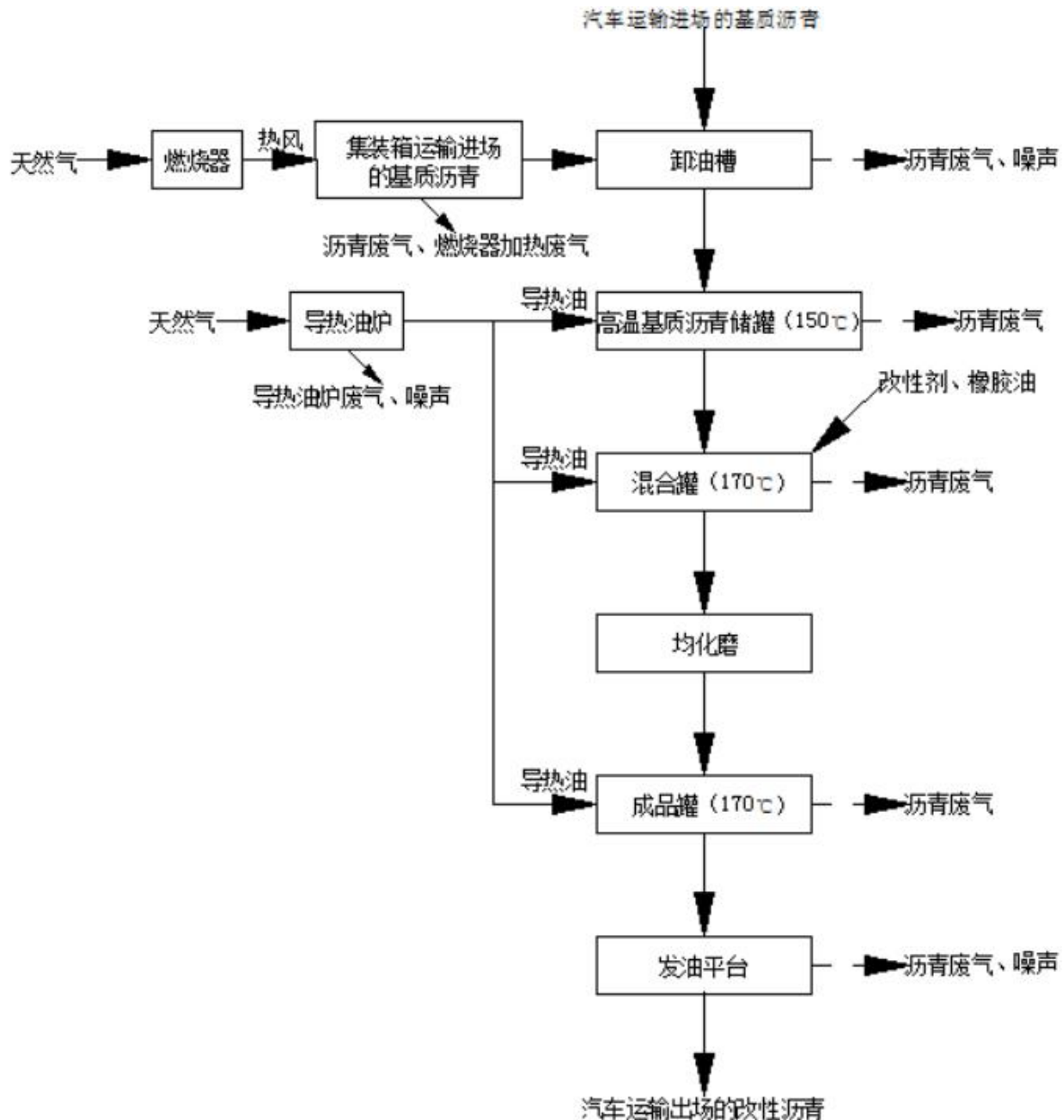
图 2.2-2 改性沥青、彩色沥青、橡胶沥青生产工艺及产污环节图
