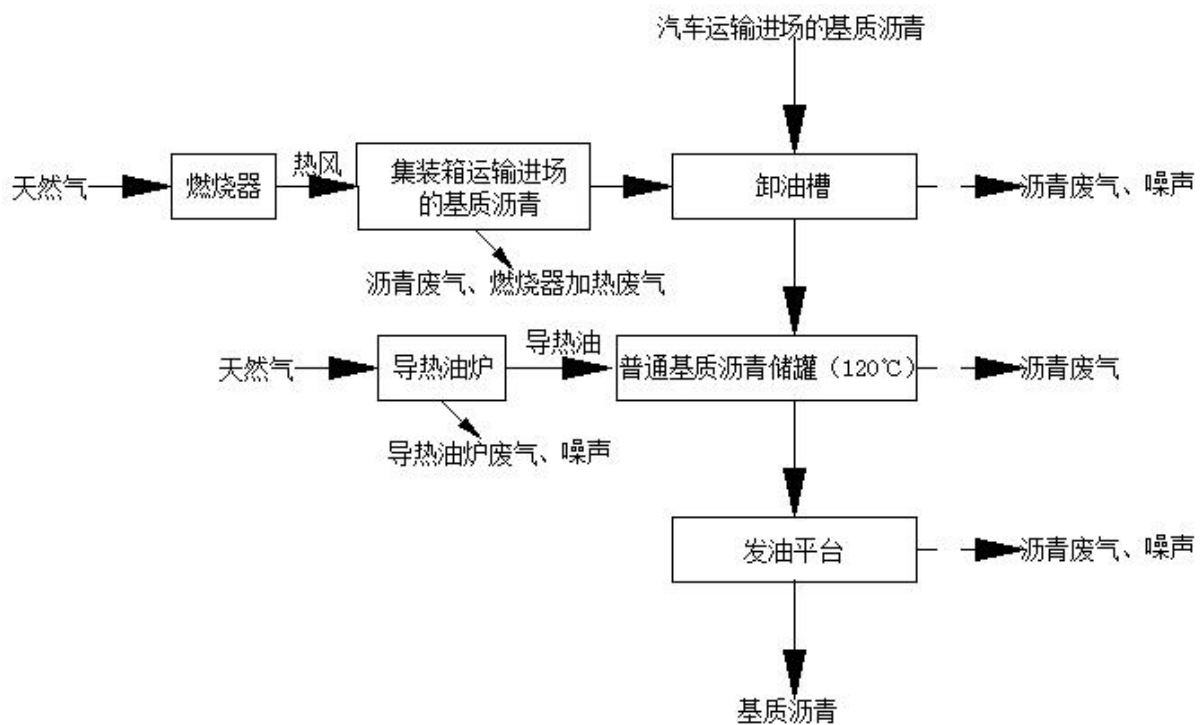
图 2.2-1 基质沥青的产污环节图
