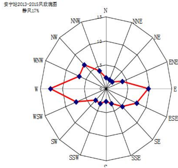
图 2.1.3-1 安宁风玫瑰图
